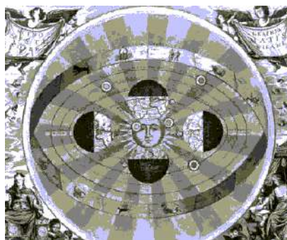
Sistema de Copérnico
